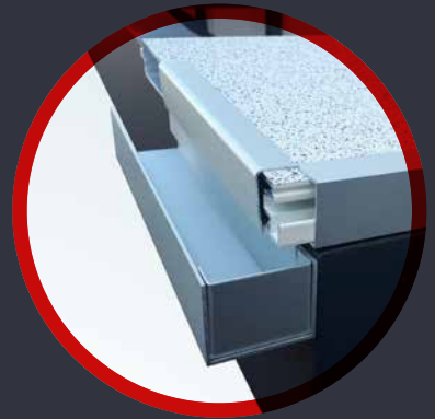
Regenrinne Balk.0010e
